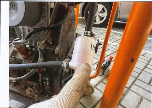
102-S008-03-柴油濾清器檢查
